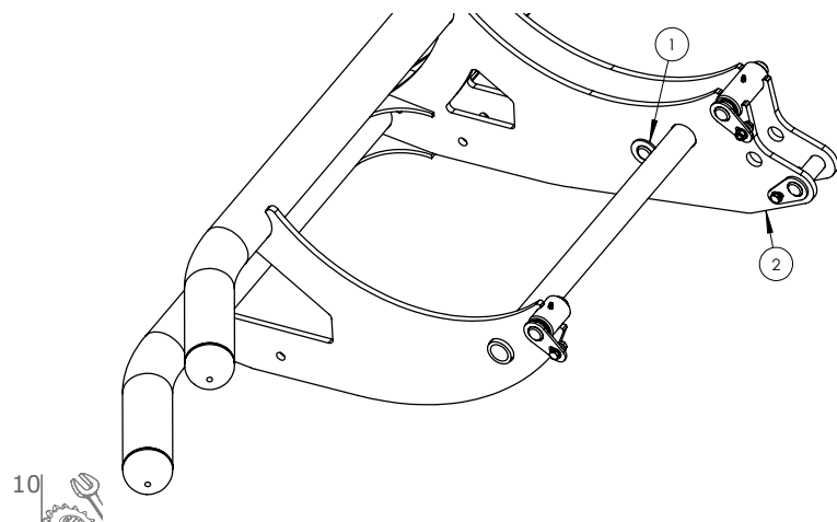
III. 4.2 Goupille de sécurité du bras de chargement ; position de travail
